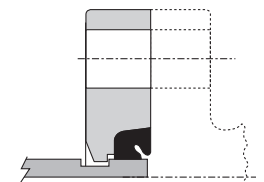
9 FLANGE
