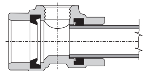
6 SOCK-IT®
