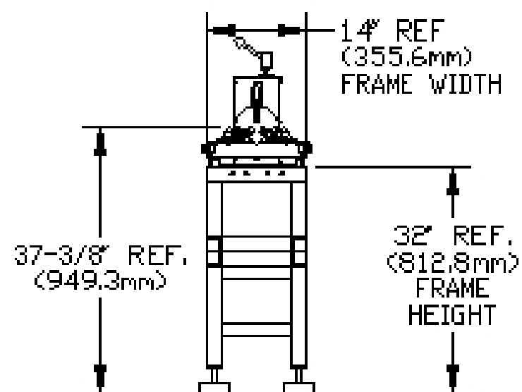
RIGHT END ELEVATION
